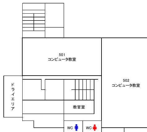
地下1階
